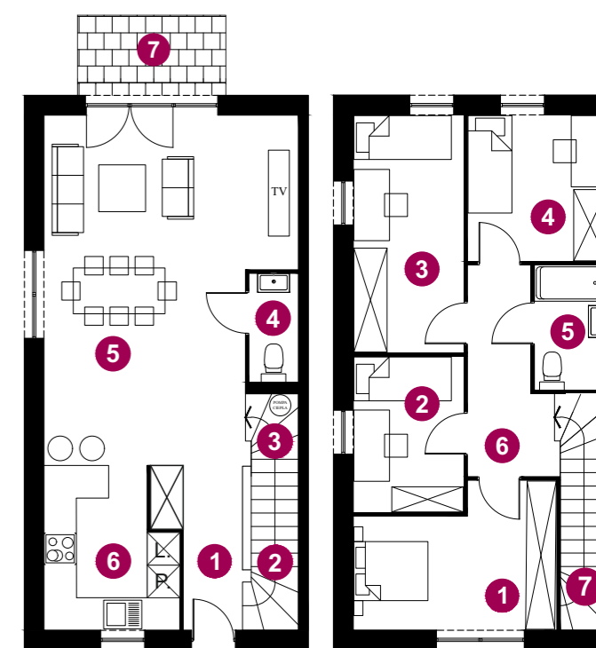
RZUT PARTERU
